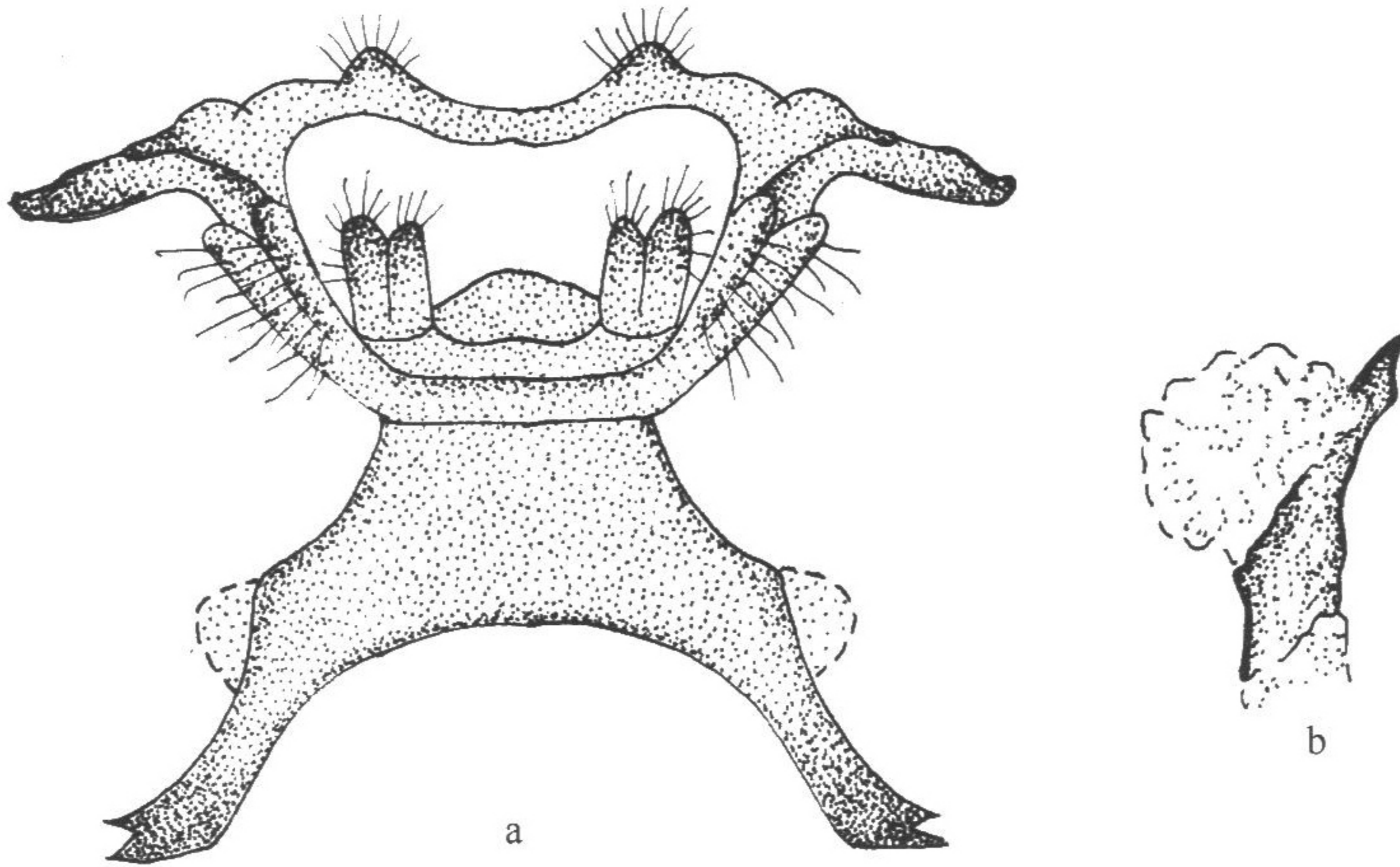
图 80 打箭杂枯叶蛾 Kunugia tamsi tamsi (Lajonquiere)
